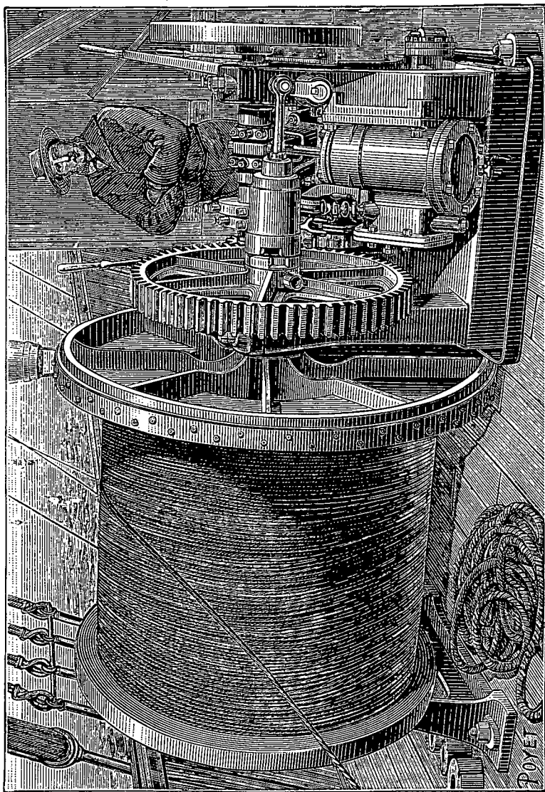
Fig. 17. — Treuil pour enrouler le câble d'acier (l'après une photographie).
