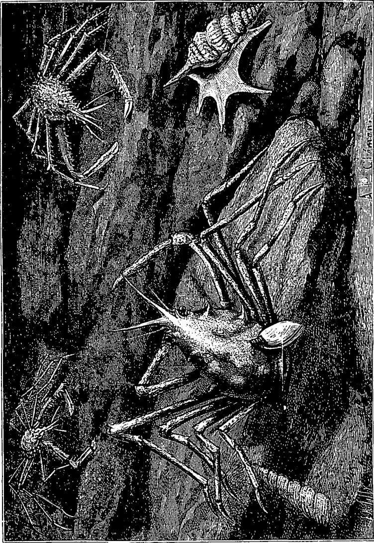
Fig. 38. — Sycramathia Carpentieri (A. M.-Edw.). — Au second plan, Eryastrius Clouei (A. M.-Edw.) et Lispognathus Thomsoni (A. M.-Edw.). 700 mètres de profondeur.
