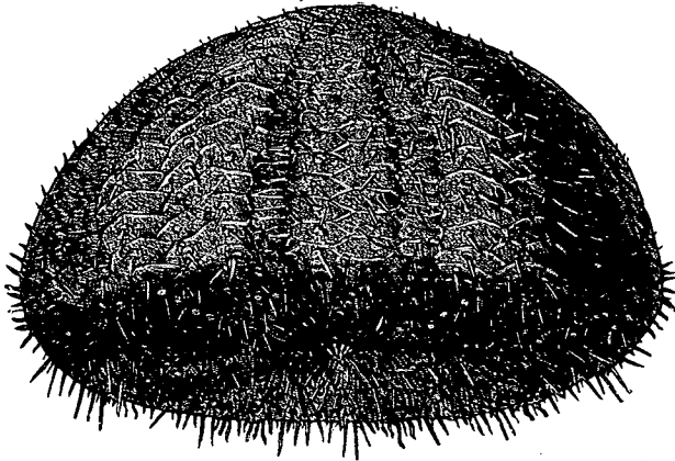
Fig. 72. — Calveria hystrix (W. Thomp.), 2,000 mètres de profondeur.
