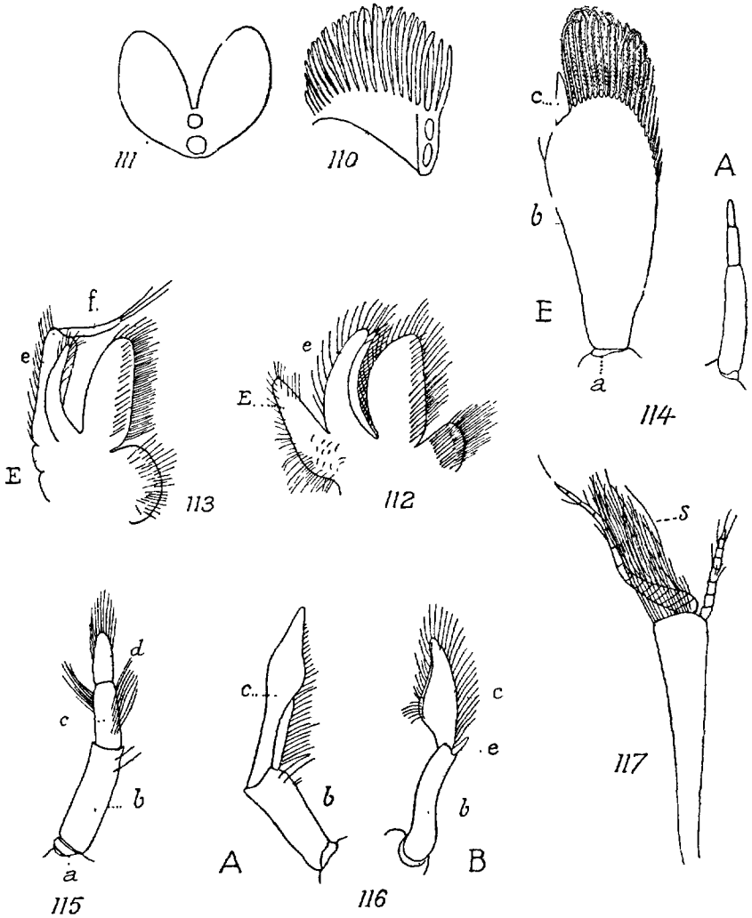
FIG. 110 à 117. — Quelques caractères des Galatheaidea : 110, trichobranchie d' Aeglea ; 111, un couple de lames phyllobranchiales de Munidopsis Sijsbeii ; 112, maxp du même ; 113, maxp avec fouet f d' Uroptychus nitidus concolor ; 114, pléopode non sexuel du ♂ A dans Munidopsis rostrata et B dans Munida Stimpsoni ; 115, pléopode femelle de Munidopsis spinosa ; 116, pléopodes 1 (A) et 2 (B) dans un ♂ de Munidopsis Antonii : a coxa, b basis, c endopodite, e exopodite ; 117, extrémité d'une antenne avec ses soies accessoires dans Munida affinis (d'après MILNE-EDWARDS et BOUVIER, 1894 b).
