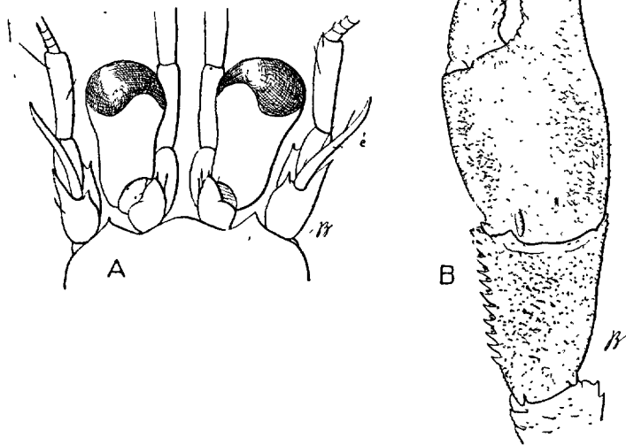
FIG. 100 bis. — Anapagurus laevis : A, front et appendices céphaliques ; B, extrémité du chélicèpe droit (d'après BOUVIER, 1896 b).
