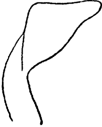
FIG. 170. — Xantho floridus , extrémité de l'endopodite de mzp^2 droit (d'après BOUVIER 1898).
