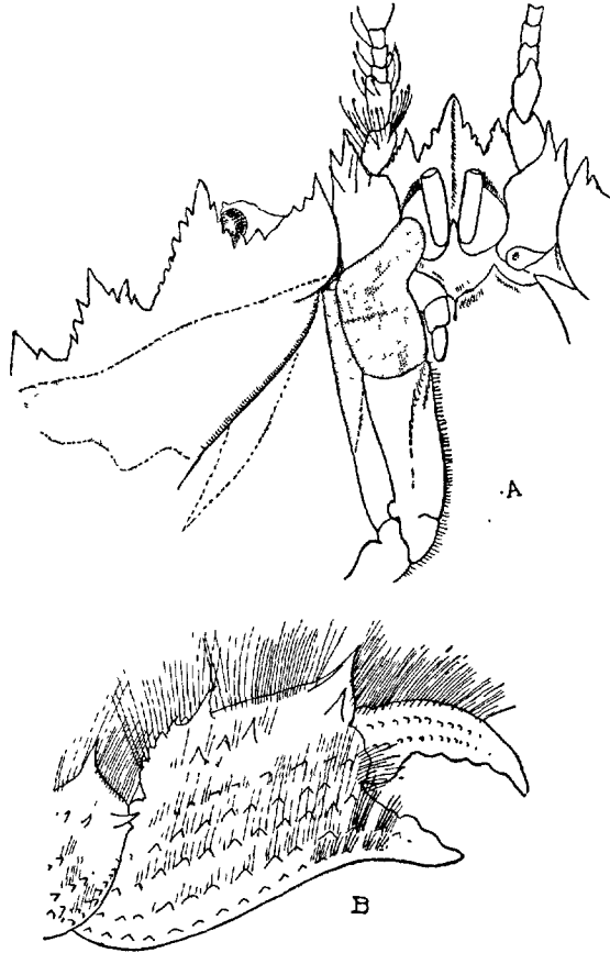
FIG. 147. — Atelecyclus rotundatus : A, appendices céphaliques et cadre buccal où l'on n'a laissé en place que mzp , face inférieure ; les parties en grisé sont partout recouvertes d'une toison de longs poils (Le pléopode I du ♂, en baguette droite, s'avance presque jusqu'à la base de mzp ) ; B, pince droite du ♂, face externe (original).
