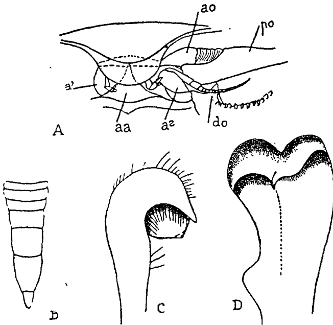
FIG. 177. — Uca Tangeri : A, rapports du front qui se rabat sur les antennules a^1 et l'arceau antennulaire aa recouvrant en partie l'arceau oculaire ao , base du pédoncule oculaire gauche po ; antenne a^2 de même côté, do dent infra-orbitaire interne ; B, abdomen du ♂ ; C, extrémité du pléopode 1 vue de côté et D, la même vue en dedans (original).
