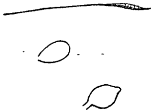
FIG. 209. — Rochinia Carpenteri : petits poils papilliformes qui figurent de fins granules à la surface du test — et poil plus long à lancette denticulée du cou (original).
