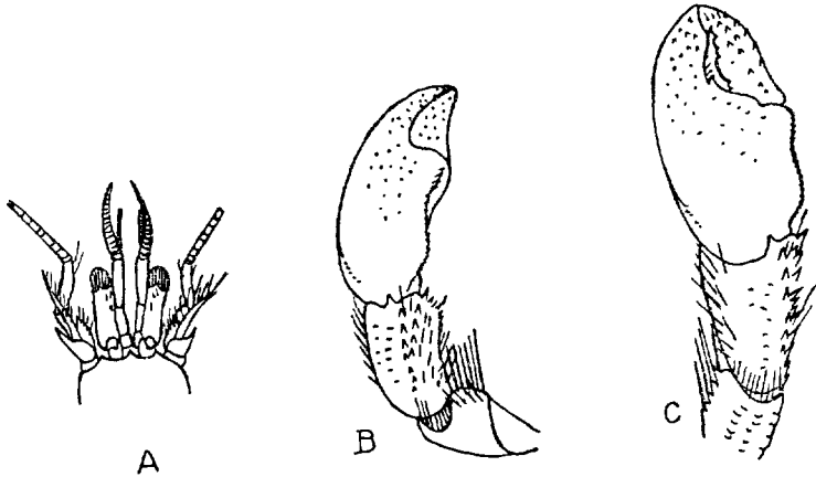
FIG. 97. — Eupagurus Chevreuxi : A front et appendices céphaliques ; B extrémité du chélimpède droit vu obliquement en dedans et C vue en dessus (BOUVIER, 1896 b.)
