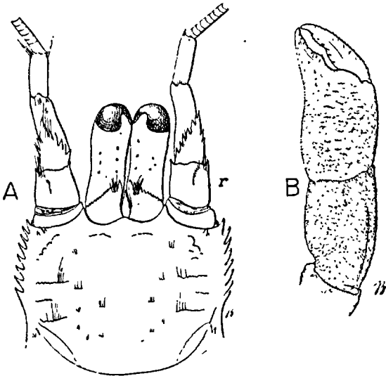
FIG. 81. — Diogenes pugilator : A, région antérieure de la carapace avec po et a 2 ; B, chélopède droit (d'après BOUVIER, 1896 b).
