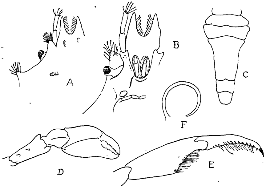
FIG. 211. — Acanihonyx lunulatus : A, rostre et région frontale gauche en dessus ; B, région frontale droite en dessus ; C, abdomen du ♂ ; D, chélicèpe droit ; E, propode et doigt de p 5 , face externe ; F, un poil en crochet (original).
