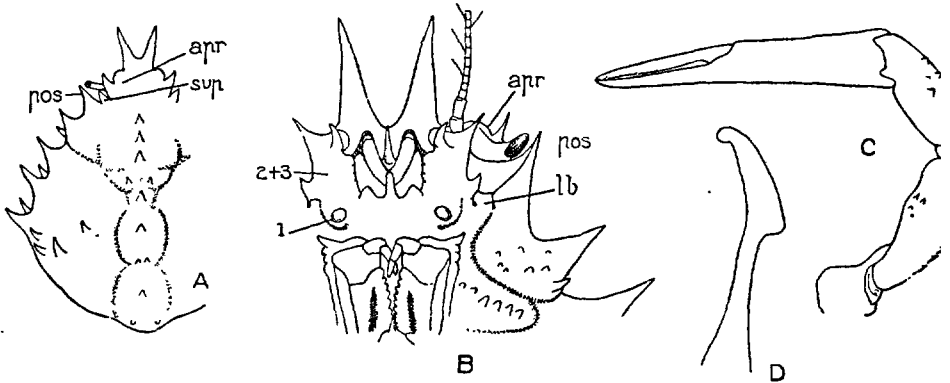
FIG. 195. — Maia squinado ♂ : A, face dorsale de la carapace et B, région fronto-buccale en dessous ( apr auvent préorbitaire, pos pointe postorbitaire, sup épine supra-orbitaire, lb lobe intra-orbitaire, 1 tubercule urinaire, 2 + 3 grand article basal des pédoncules antennaires) ; C, chélicèpe gauche ; D, extrémité du pléopode 1 droit (original).
