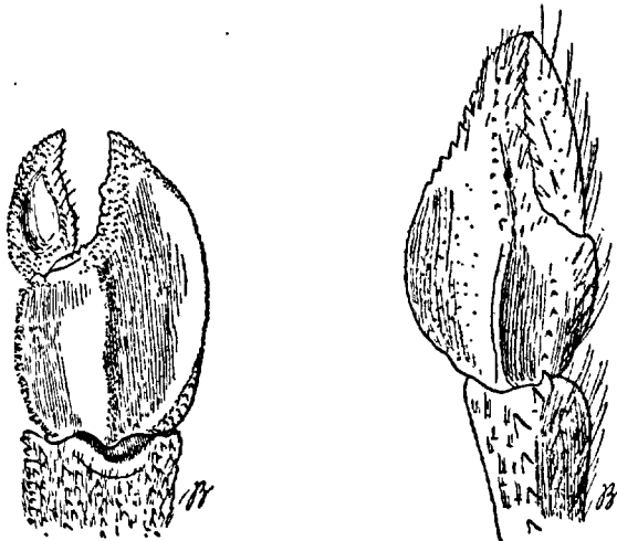
FIG. 89-90. — Eupagurus excavatus : extrémité des chélicères, face dorsale: 89, du chélicère droit; — 90, du chélicère gauche (d'après BOUVIER, 1896 b).
