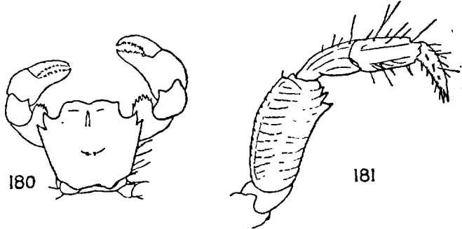
FIG. 180-181. — 180. Pachygrapsus maurus , exemplaire avec ses chélicépes (d'après LUCAS, 1849). — 181. Pachygrapsus transversus , patte postérieure droite (original).
