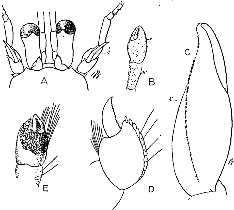
FIG. 103. — Anapagurus curvidactylus : A, front et appendices céphaliques ; B, extrémité du chélicède droit ; C, pince droite vue obliquement en dehors pour montrer la série c de denticules du bord externe ; D, extrémité de p^4 droit face externe ; E, même face de p^4 (d'après BOUVIER, 1896 b).
