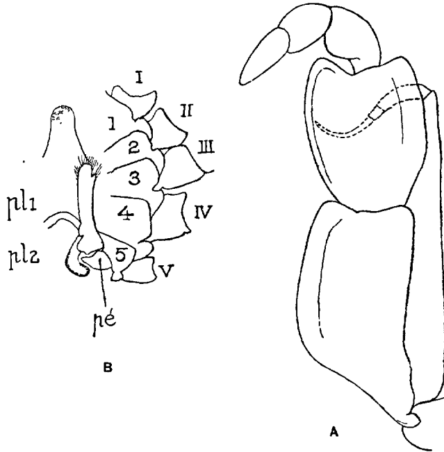
FIG. 186. — Eriocheir sinensis : B, sternites thoraciques (I à V) avec la base des pattes correspondantes (I à V), le pénis pé et les pléopodes sexuels gauches pl^I et pl^II ; A, mzp^I gauche (original).
