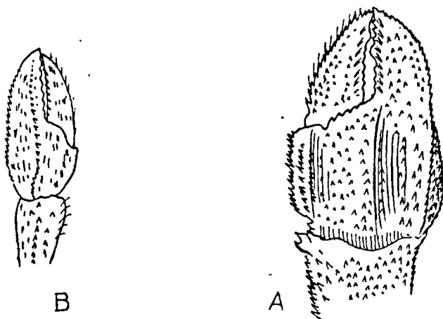
FIG. 91. — Eupagurus variabilis ; extrémité des chélicères : face dorsale, A, du chélicère droit, B, du gauche (d'après BOUVIER, 1896 b).
