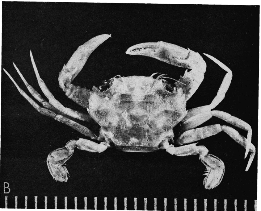
A, Thalamita philippinensis , new species, holotype. B, T. pseudopoissoni , new species, holotype. (Scale 1 mm.)
